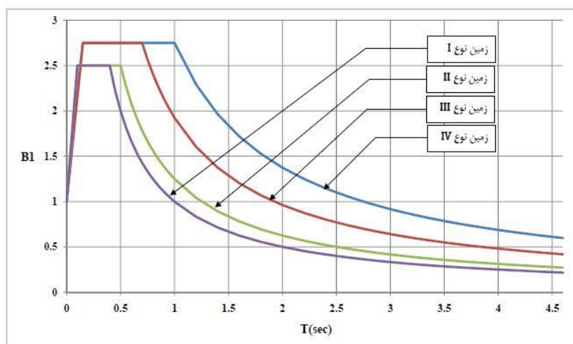
شکل ۲-۱-ب- ضریب شکل طبق طرح برای انواع زمین‌های مندرج در بند (۲-۴) با خطر زیاد و خیلی زیاد
